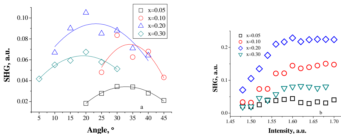
Рис. 1. Кутова та енергетична залежність генерації другої гармоніки у монокристалах твердого розчину \text{AgGaGe}_{3(1-x)}\text{Si}_{3x}\text{Se}_8
