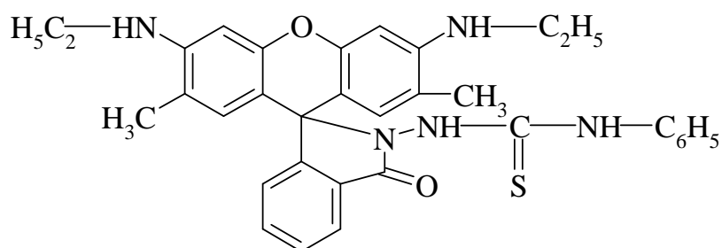
Рис. 1. Формула 1-[3', 6'-біс(етиламіно)-2', 7'-диметил-3-оксо-2,3-дигідроспіро[ізоіндол-1,9'-ксантен]-2-іл]-2-фенілтіосечовини.
