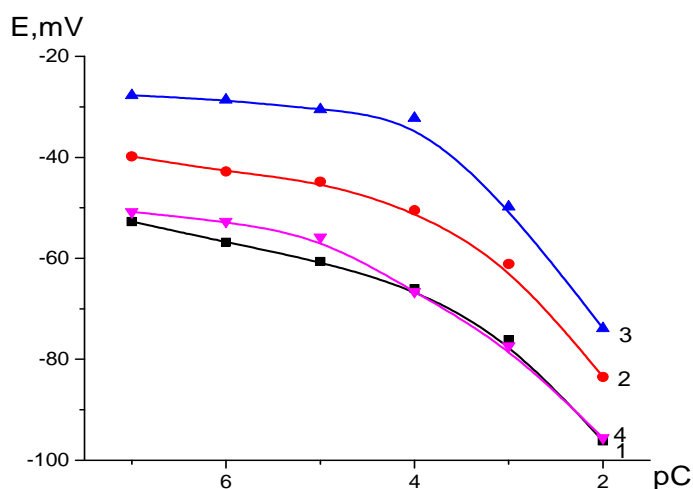
Рис. 1. Вплив кількості ЕАР на калібрувальні залежності ІСЕ з мембраною на основі родаміну б Ж, пластифікованою ДБФ.
