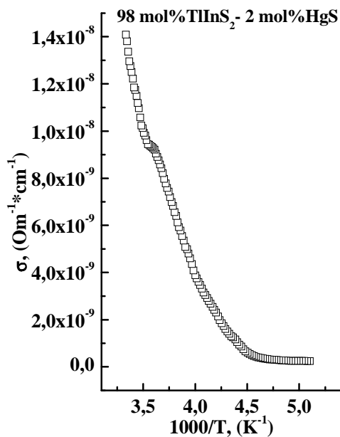
Рис. 1. Температурна залежність питомої темної електропровідності кристала 98mol%TlInS 2 -2mol%HgS
