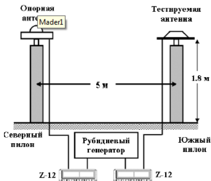
Рис. 2 Установка для абсолютного калибрования антенн в реальном времени
