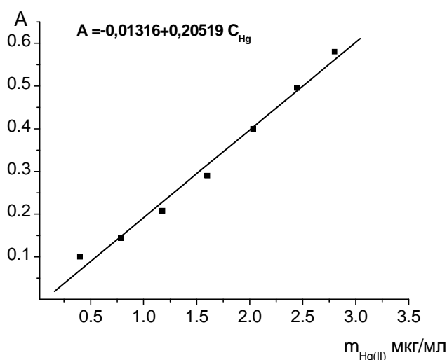
Рис 2. Градувальний графік; \text{pH}=4 ; C_{\text{Hg(II)}} = 4 \cdot 10^{-5} моль/л; \text{pH} = 4 ; C_R = 2 \cdot 10^{-4} моль/л; l = 1 см;
