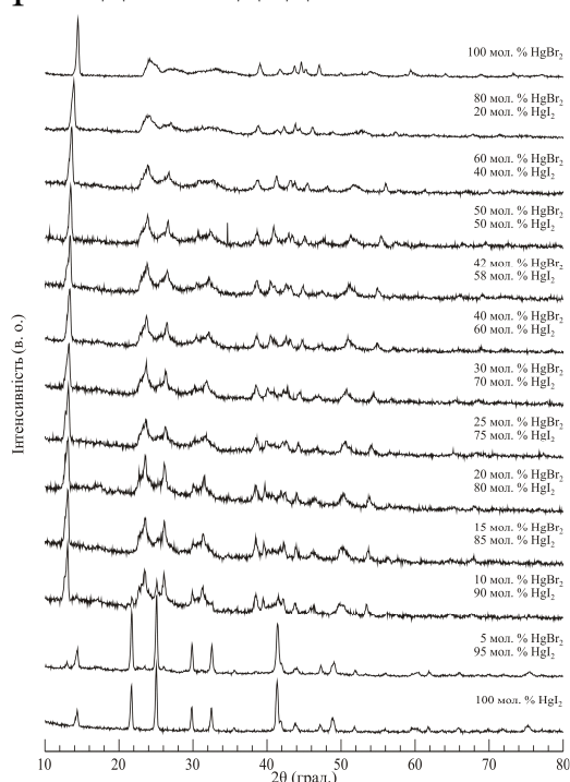
Рис. 1. Дифрактограми зразків системи HgI_2-HgBr_2
