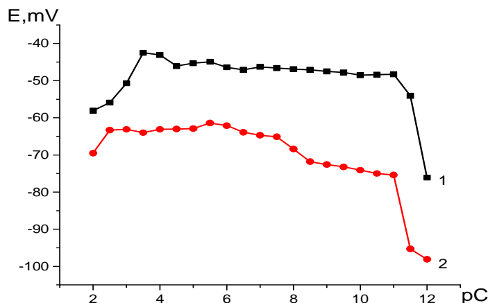
Рис. 2. Вплив рН розчину на роботу сенсора на основі ІА сахарину з родаміном С із складом: ЕАР – 4%, ДОФ – 67% (1 – рС = 4, 2 – рС = 3).
