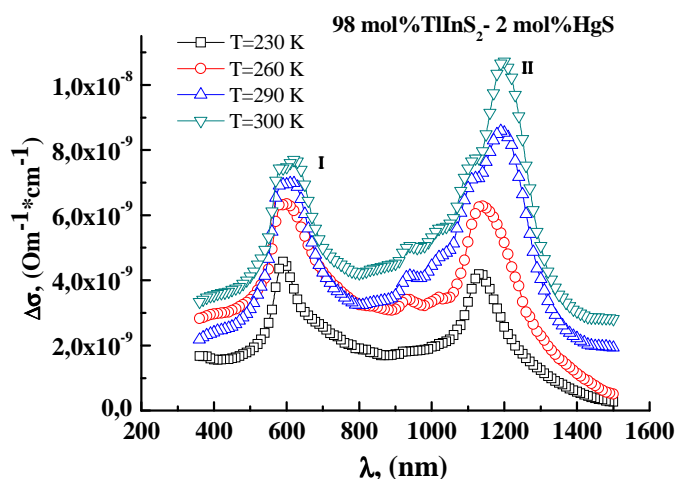
Рис. 2. Спектральний розподіл фотопровідності кристала 98\text{mol}\% \text{TlInS}_2 - 2\text{mol}\% \text{HgS}
