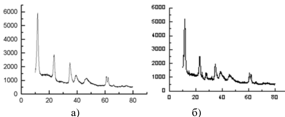
Рис. 1. Рентгенограма Mg-Al-CO 3 гідроталькіту, синтезованого методом осадження з розчинів нітратів (а) та хлоридів (б) магнію і алюмінію (Mg : Al = 3:1)
