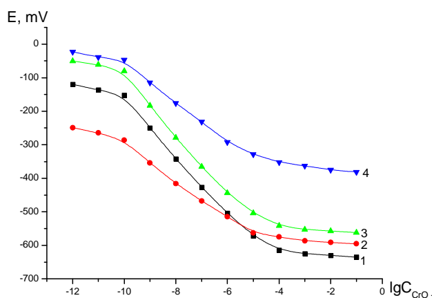
Рис. 2. Залежність потенціалу електродів на основі Mg-Al-CO 3 гідроталькіту від концентрації хромат-іонів (CrO 4 2- )
