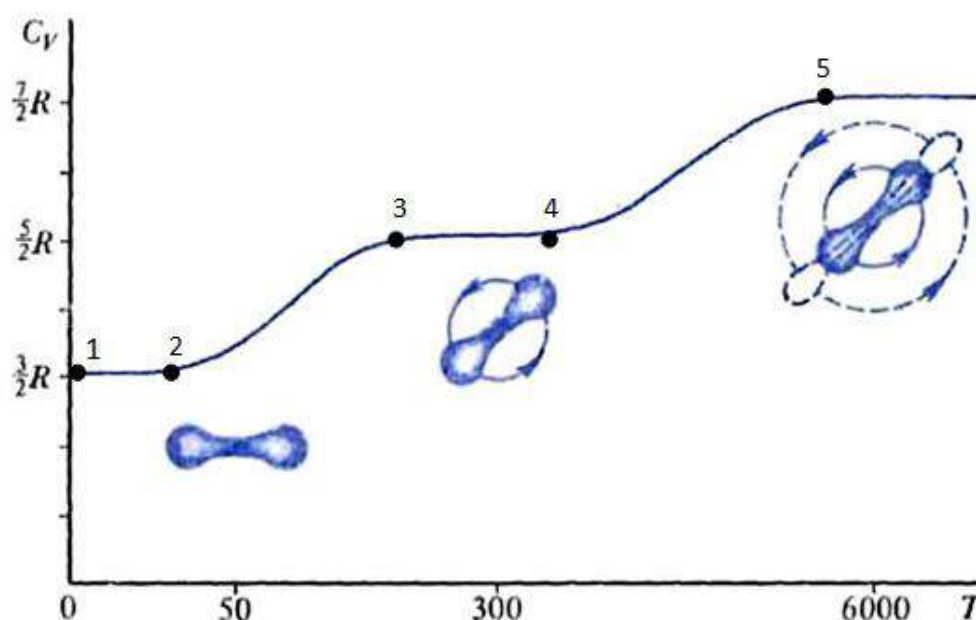
Рис. 1. Експериментальна залежність молярної теплоємності молекулярного водню від температури
